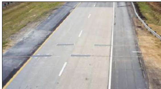
Εικόνα 4.7 Σύστημα μέτρησης κυκλοφορίας WIM σε δύσκαμπτο οδόστρωμα
