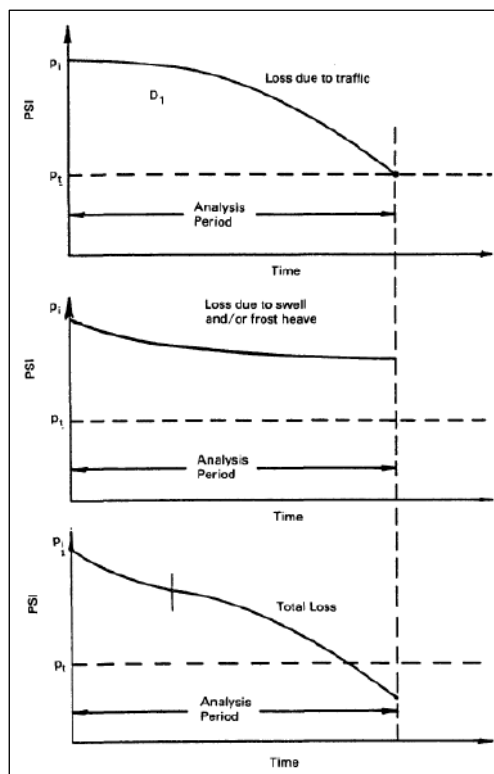
Εικόνα 3.13 Απώλεια εξυπηρετικότητας οδοστρώματος σε συνάρτηση με το χρόνο κατά AASHTO93 [AASHTO, 1993]
