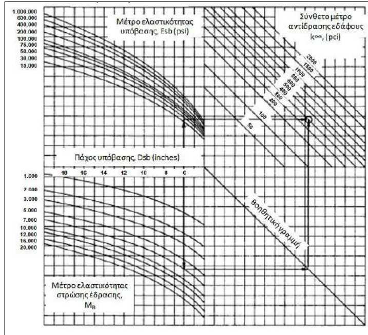
Εικόνα 3.14 Υπολογισμός σύνθετου μέτρου αντίδρασης εδάφους k_{eq} σε περίπτωση που υφίσταται στρώση υπόβασης κατά AASHTO93 [AASHTO, 1993]
