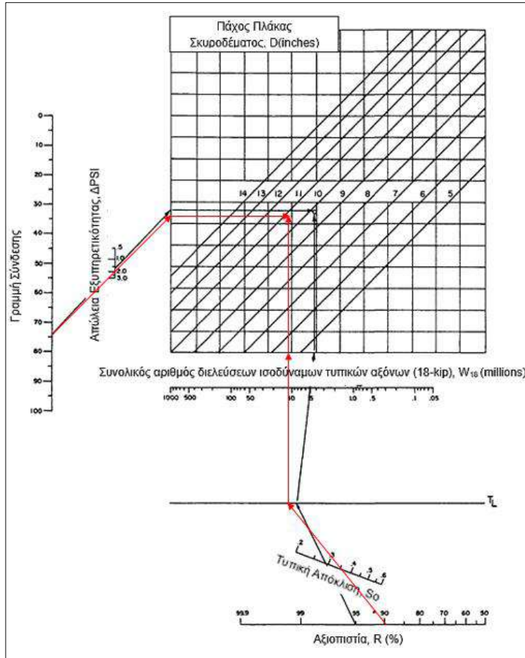
Εικόνα 5.3B Υπολογισμός πάχους πλάκας σκυροδέματος με τη μέθοδο AASHTO93 (συνέχεια από 5.3α)
